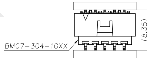
MATEING VIEW SCALE 1:2
